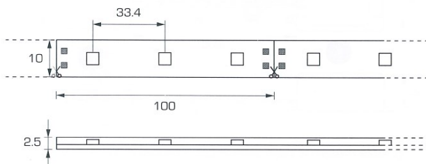
LED's auf flexiblem 5m Band, selbstklebend
