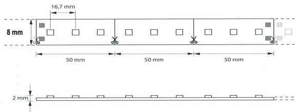
LED's auf flexiblem 6m Band, selbstklebend
