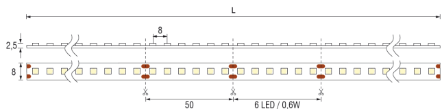
LED's auf flexiblen 5m Band, selbstklebend
