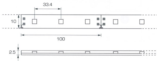
LED's auf flexiblen 5m Band, selbstklebend
